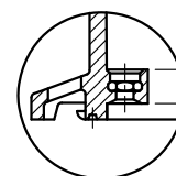
M4 ボス部 詳細図
